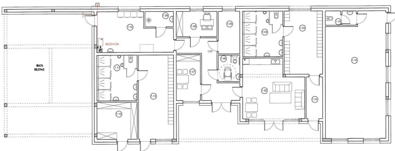
Rysunek 4. Rzut parteru budynku zaplecza boiska sportowego.
