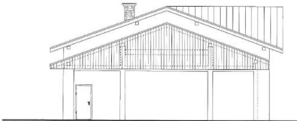
Rysunek 3. Elewacja południowo-wschodnia.
